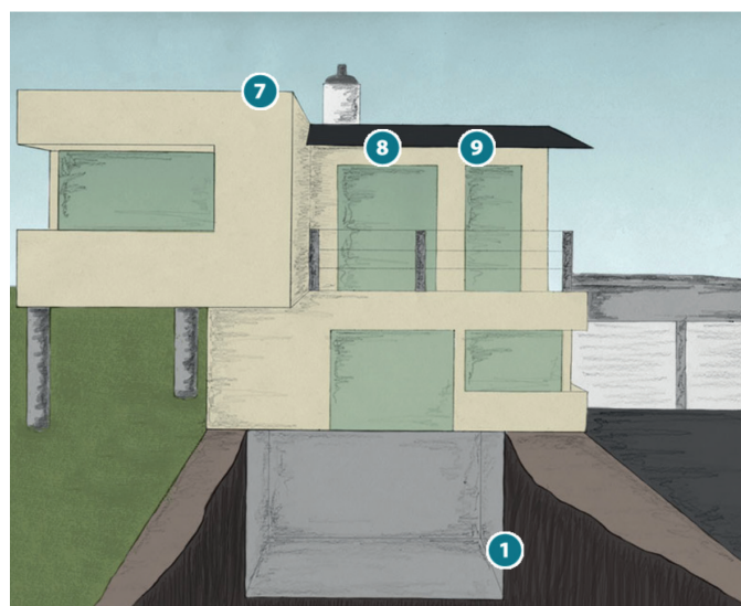
1_Abdichtung Kelleraußenwand, 7_Schutz Bitumendachbahn, 8_Abdichtung Dachrinne, 9_Abdichtung Anschlussbereich
